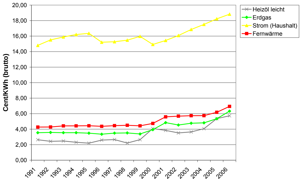
Abbildung 9: Spezifische Energiepreise in Cent/kWh [BMW 2007]
