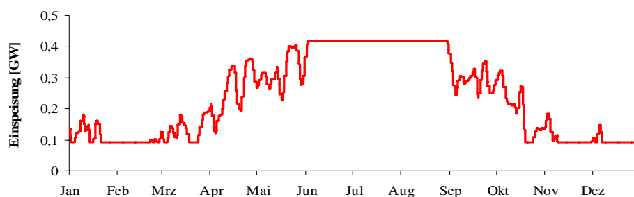
Abbildung 3-8: Simulierte Einspeisung wärmegeführter Geothermieanlagen des Jahres 2020 in stündlicher Auflösung (0,4 GW) (temperaturbereinigt). Quelle: eigene Berechnungen nach BEE-Szenario.
