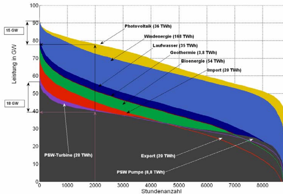
Abbildung 6-4: Jahresdauerlinien mit der Stromerzeugung der einzelnen EE-Quellen. Quelle: eigene Berechnungen nach BEE-Szenario.
