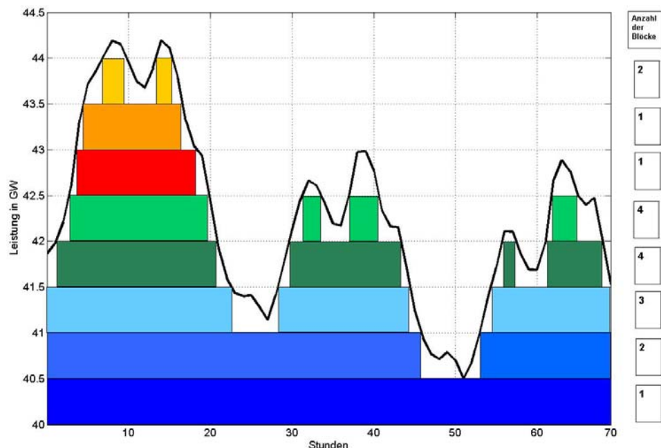
Abbildung 6-6: Exemplarische Veranschaulichung der Häufigkeit der An- und Abfahrvorgänge von 500 MW Kraftwerksblöcken im Leistungsreich von 40 GW bis 44 GW für einen Zeitraum vom 70 Stunden. Quelle: eigene Darstellung.
