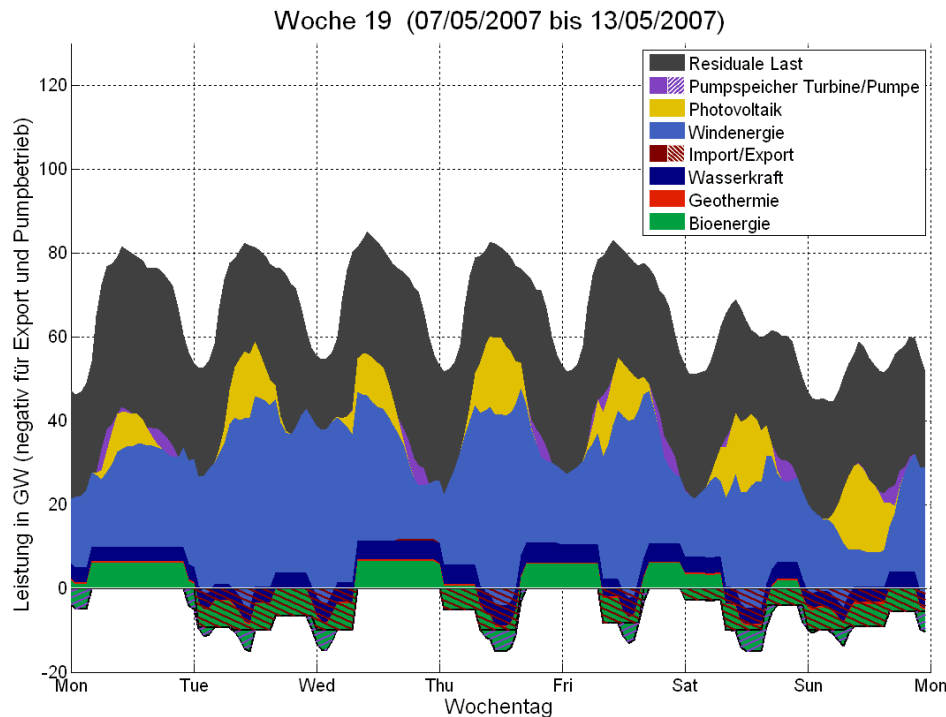
Abb. 5: Woche mit dem Moment der maximalen EE-Einspeisung (2020)
