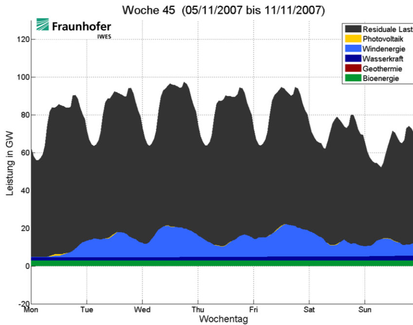
Abb. 8: Woche mit dem Moment der Jahreshöchstlast (2007)
