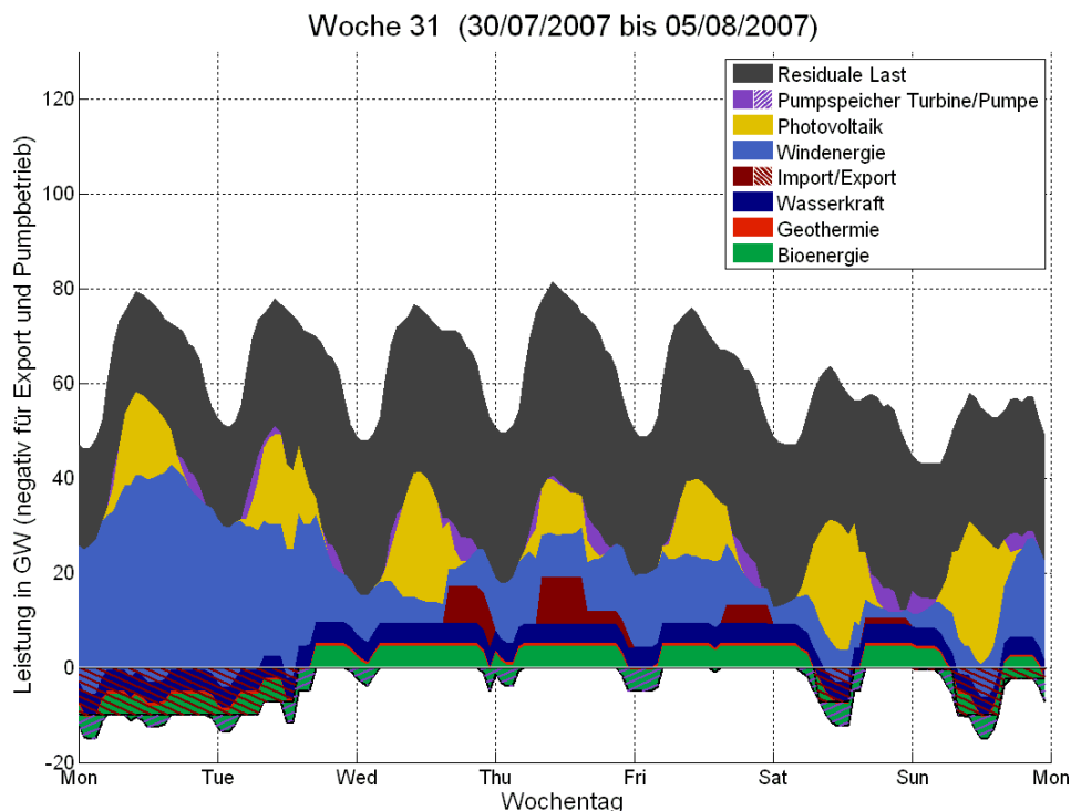
Abb. 7: Woche mit dem Moment der minimalen EE-Einspeisung (2020)
