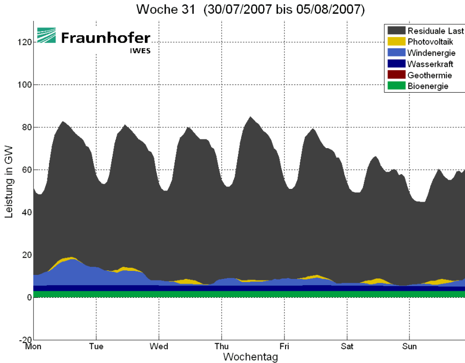
Abb. 6: Woche mit dem Moment der minimalen EE-Einspeisung (2007)
