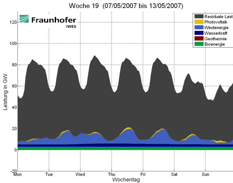
Abb. 4: Woche mit dem Moment der maximalen EE-Einspeisung (2007)
