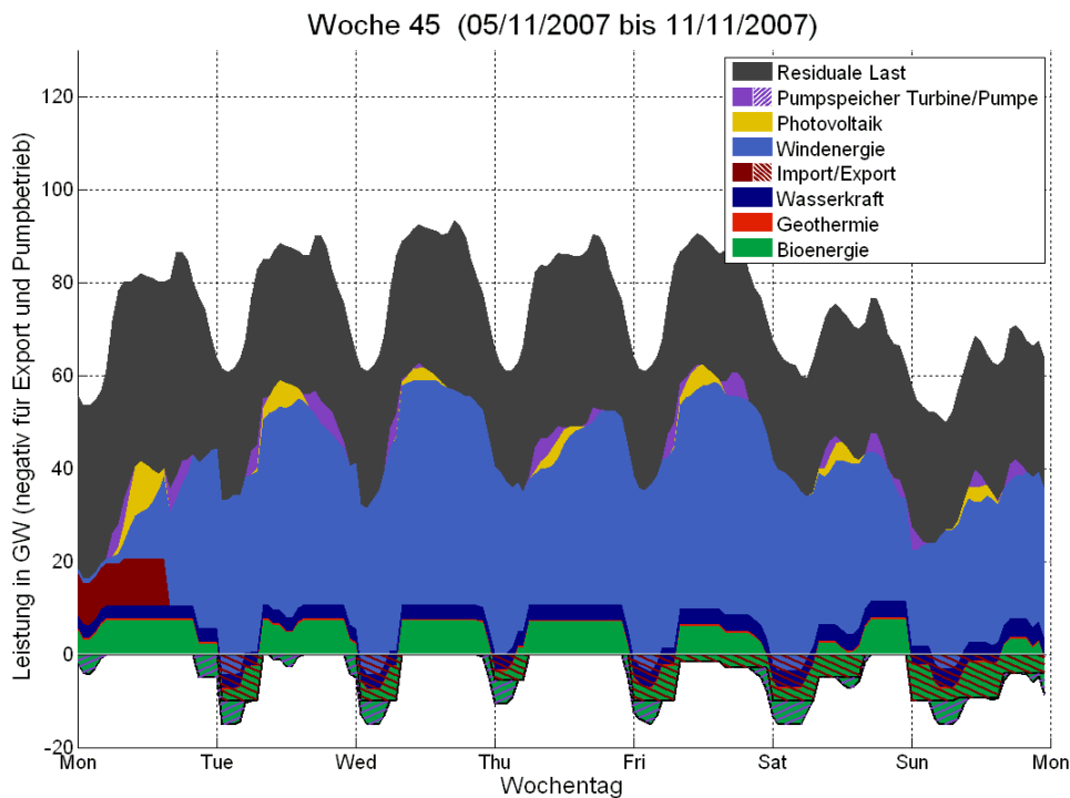
Abb. 9: Woche mit dem Moment der Jahreshöchstlast (2020)
