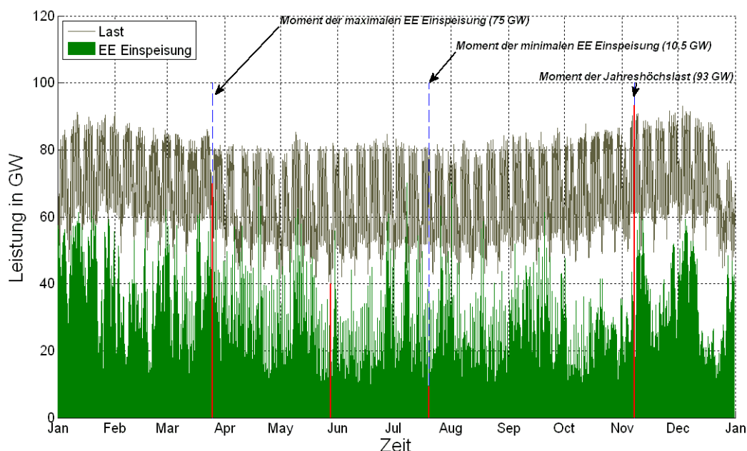
Abb. 3: Verteilung ausgewählter „Extremwochen“ im Kalenderjahr.
