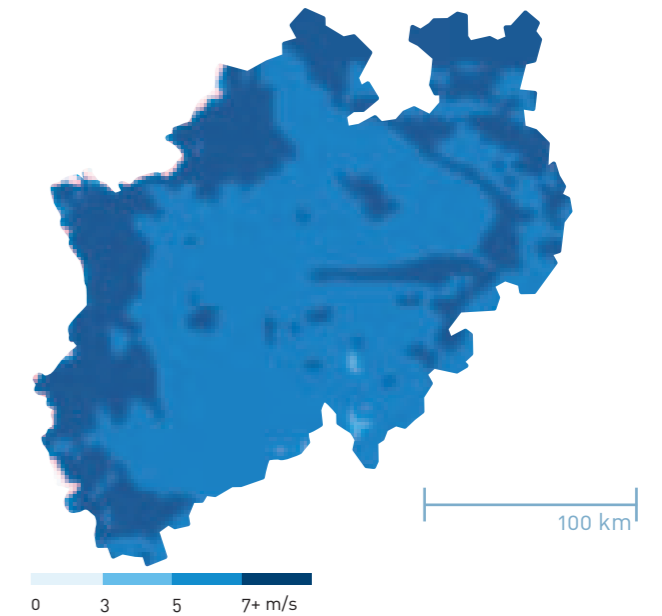
Windgeschwindigkeiten in 120 m Höhe
