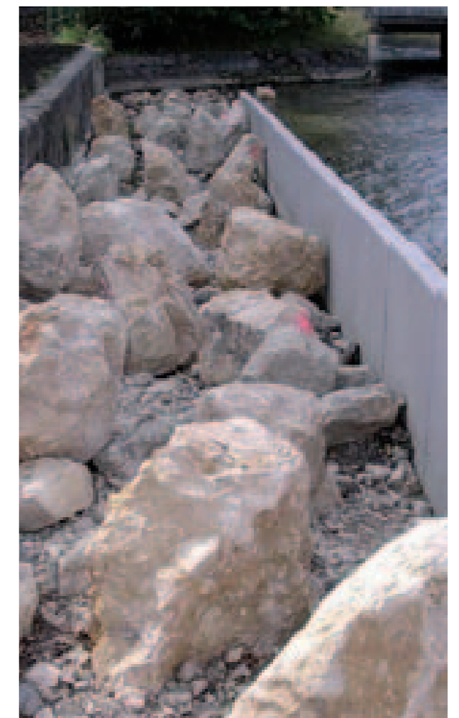
Ein aufwändiger Fischpass verbesserte die ökologische Situation der Alb.
