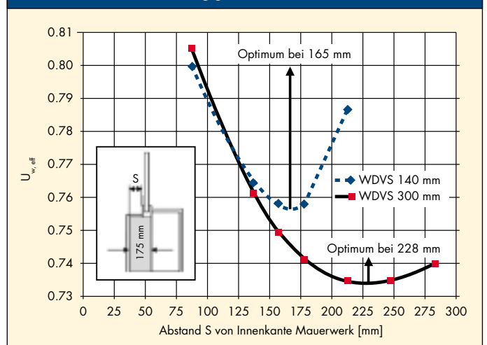
Abb 4: Berechneter Fenster- U_w -Wert für ein hochgedämmtes Fenster in Abhängigkeit der Einbausituation
