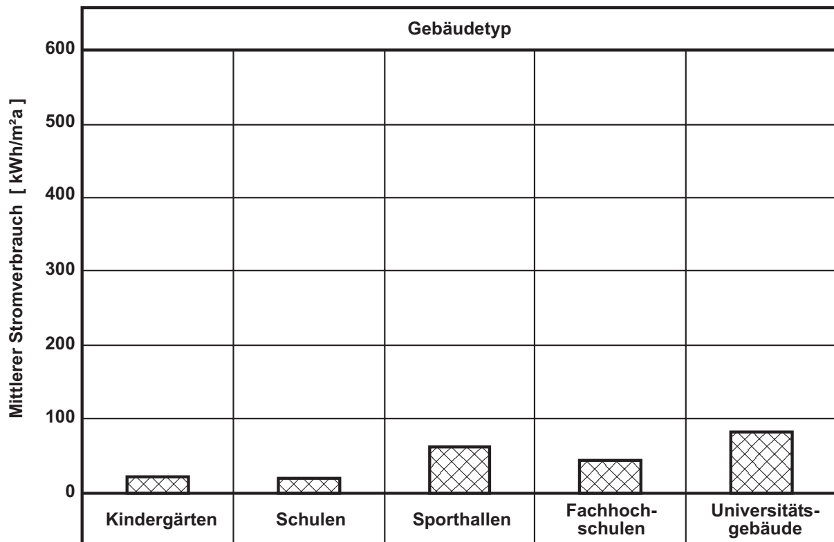
Bild 29: Mittelwerte des Stromverbrauchs der Daten innerhalb der Standardabweichung für die verschiedenen Bildungsgebäudetypen.
