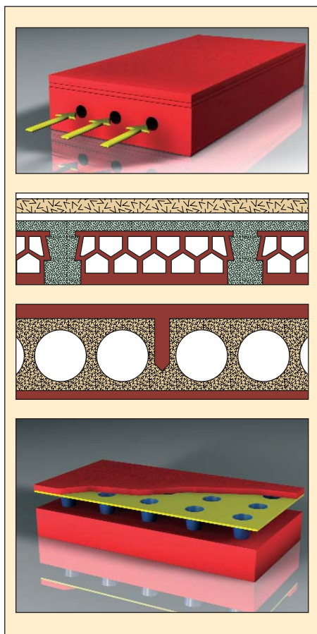
Skizzen von Hypokaustenelementen (Fertigdecken, Hohlböden, Rohrregister)
